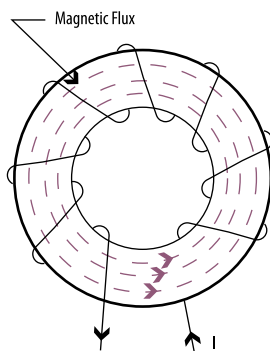
Рис. 5. Индуктор с тороидальным сердечником
