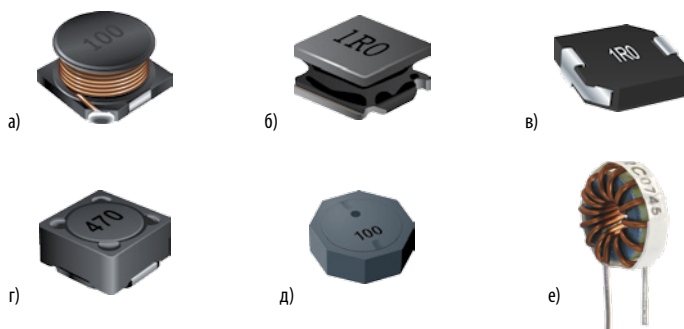
Рис. 9. Некоторые семейства катушек индуктивности Bourns: а) серия SDR; б) серия SRN; в) серия SRR; г) серия SRR; д) серия SRU; е) тороидальные катушки индуктивности J.W. Miller для монтажа в отверстия
