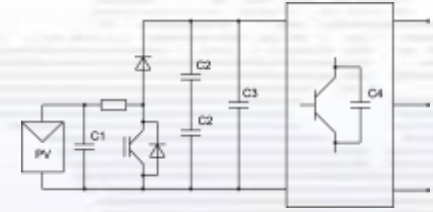
DC-Link
